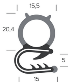
Réf : PUV019 Profil universel avec butyl 22 mm rouleau 23 m Renault premium
