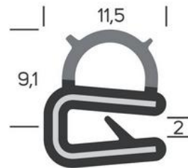
Réf : PUV006 Profil universel insert métal pour TP 11,5 mm rouleau 50 m
